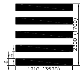
DGBB 1332 - R11
